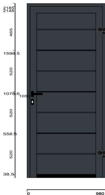
Originalskizze/Aussenansicht
